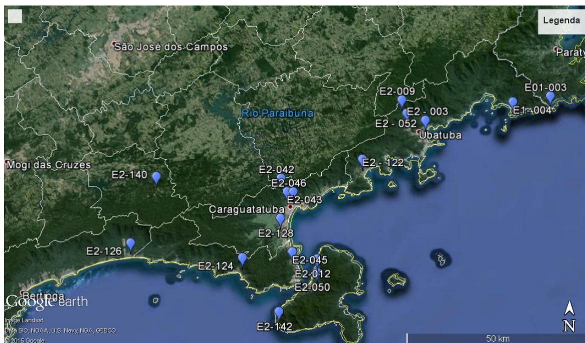
Figura 10. Localização das estações meteorológicas utilizadas no trabalho.
